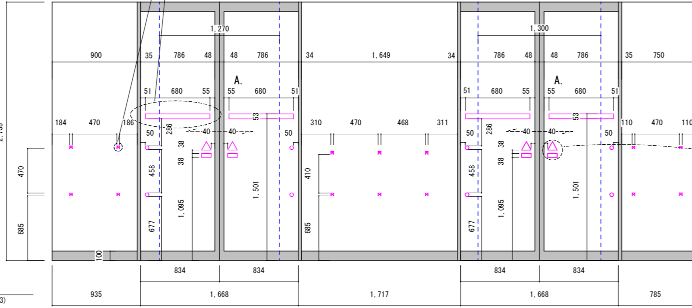
A ELEVATION Scale: 1:40 (A3)
