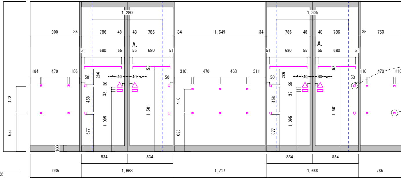
B ELEVATION Scale: 1:40 (A3)
