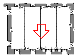
立面図④ ( ホワイエA側)
