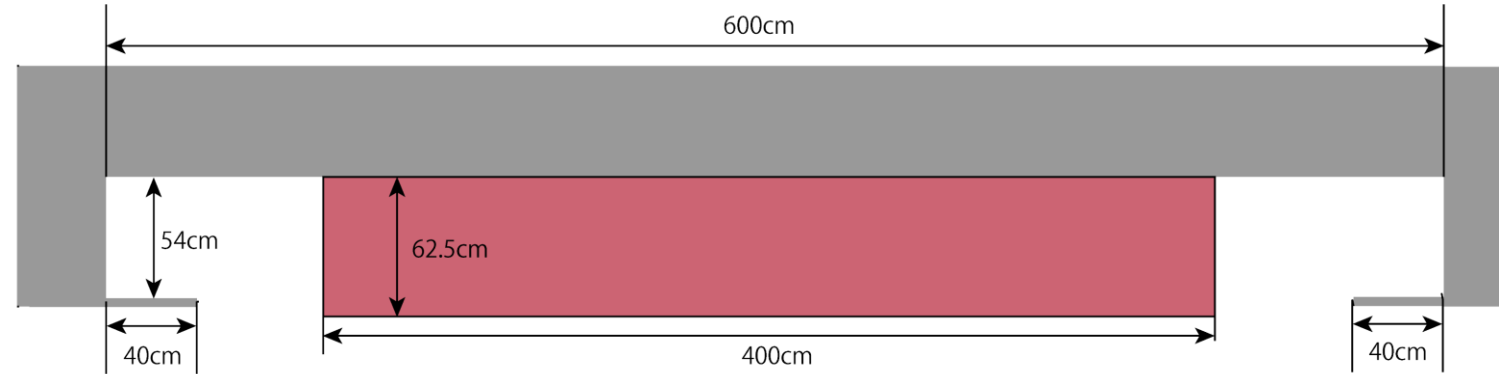
平面図
