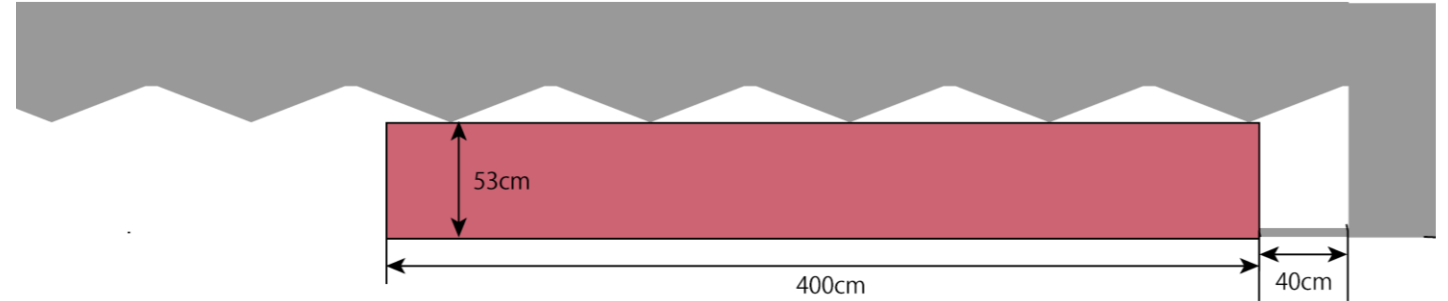
平面図
