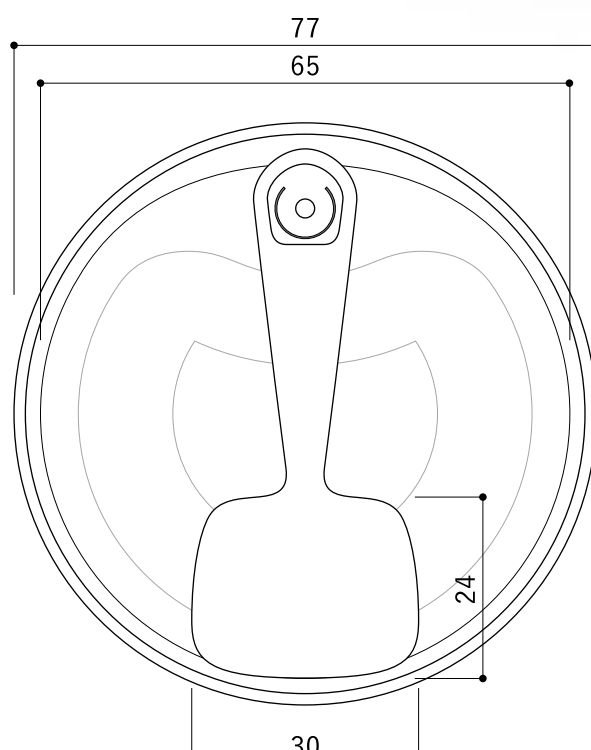
4号缶 (h113 mm) ・ 5号缶 (h81 mm) ・ 6号缶 (h59 mm) (内径 74 mm) のスプーン 1:1
