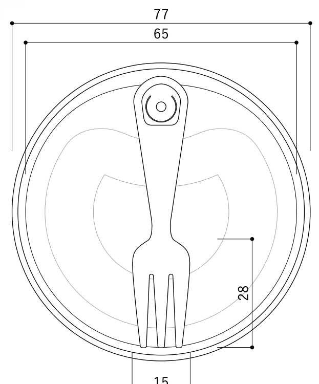
4号缶 (h113 mm) ・ 5号缶 (h81 mm) ・ 6号缶 (h59 mm) (内径 74 mm) のフォーク 1:1
