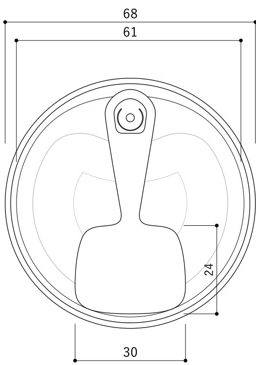
7号缶 (h101 mm) ・ 特殊7号 (h75 mm) ・ 8号缶 (h53 mm) (内径 65 mm) のスプーン 1:1
