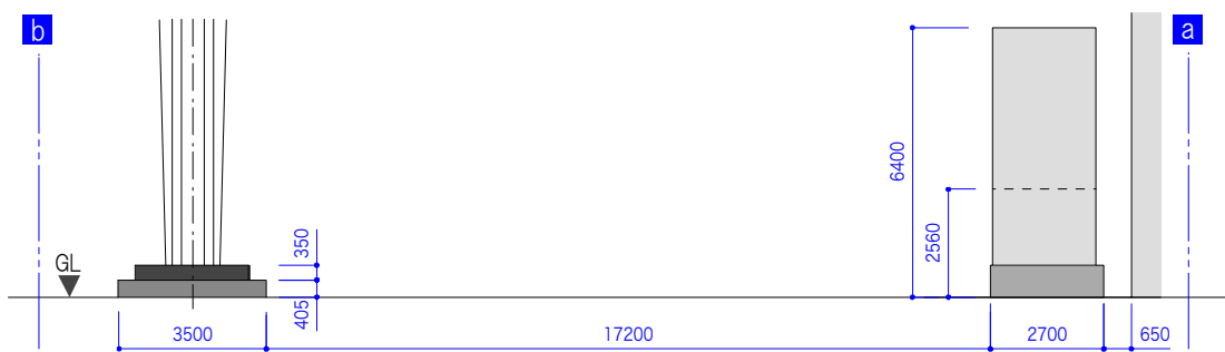
■ a-b 断面図
